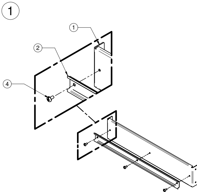
ITEM 2 RMHD - BOLT-ON DIN RAIL QTY 1
