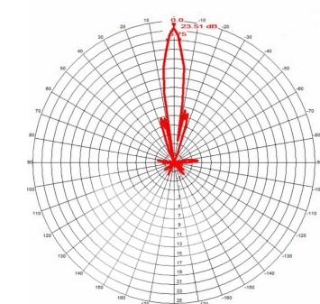
1700-2700 MHz
