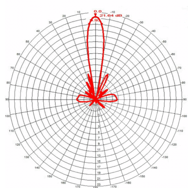
600-960 MHz
