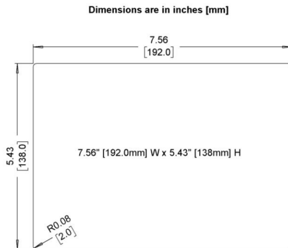
Cutout Dimensions
