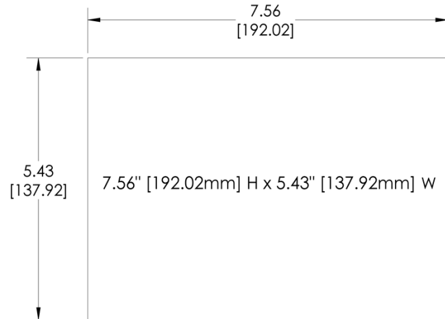
Cutout Dimensions
