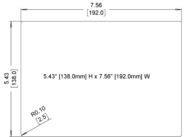
Cutout Dimensions
